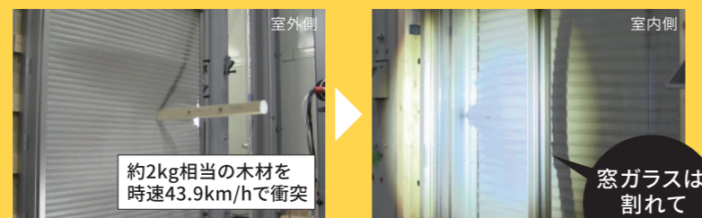
耐風シャッターGR 耐飛来物衝突性能実験
